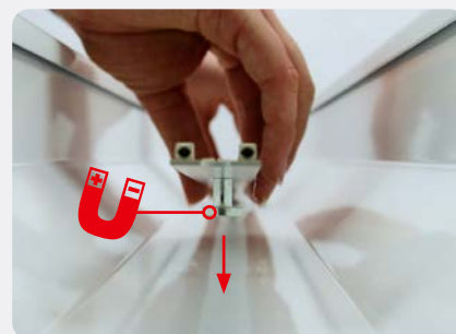
Maintien sûr du luminaire grâce à des pieds magnétiques en néodyme repositionnables.
