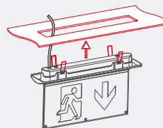
Montage au plafond, avec cadre d'encastrement
