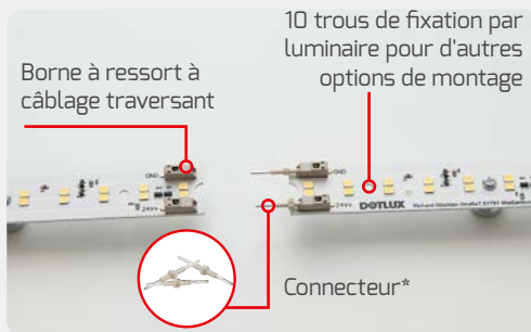
Les connecteurs à broches permettent de connecter les luminaires en série. Les sections reliées peuvent être séparées à l'aide de l'outil de déconnexion fourni.
