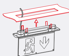
Montage au plafond, avec cadre d'encastrement
