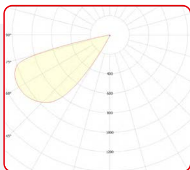
Courbe de répartition lumineuse du GUIDEround
