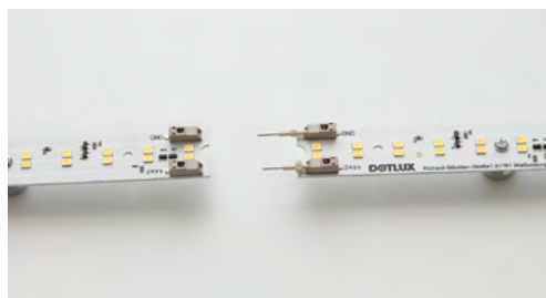
Mit Pin-Anschlüssen lassen sich die Leuchten in Reihe verbinden (inkl. Lösewerkzeug).
