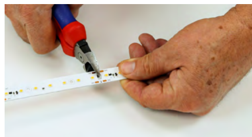
Individuell teilbar alle 10 cm; Beidseitig zwei einzelne Anschlussklemmen.
