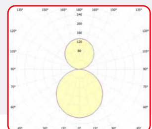
Angenehme Atmosphäre dank indirektem Lichtanteil
