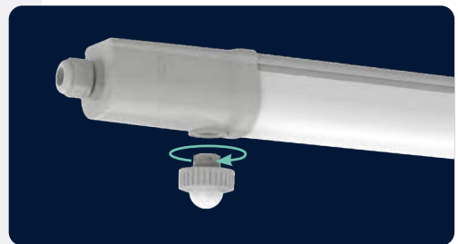
Verschlusskappe entfernen und Sensor mit TWISTLOCK eindrehen.
