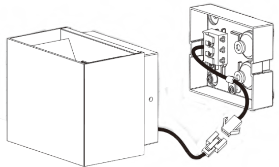
EASYbase für einfache Montage
